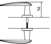
Door handles on roses
