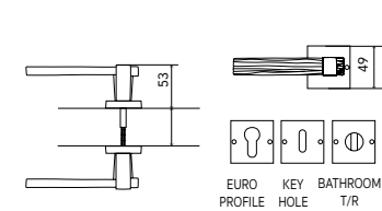
Door handles on roses
