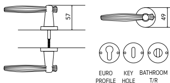
Door handles on roses
