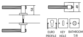
Door handles on roses
