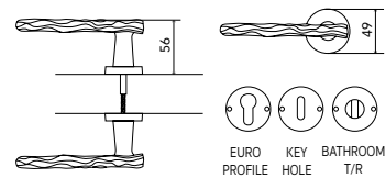
Door handles on roses
