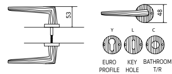
Door handles on roses
