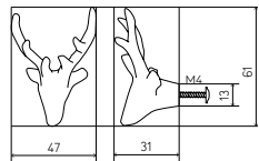
CERF Knobs
