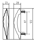
AGAVE 122 Pulls
