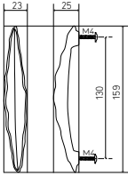
AGAVE 159 Pulls
