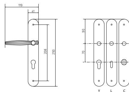
BÉQUILLE SUR PLAQUE
