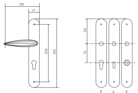
BÉQUILLE SUR PLAQUE
