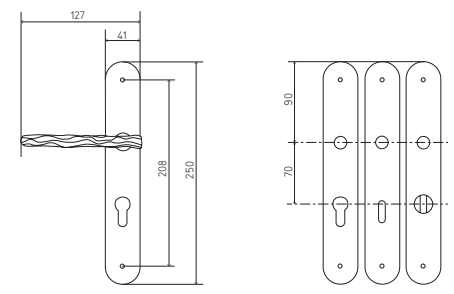
BÉQUILLE SUR PLAQUE
