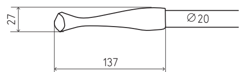
EMBOUT VIDE 20
