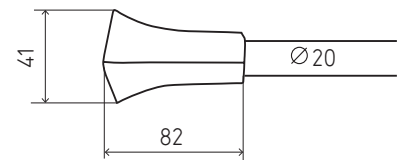
EMBOUT GARDE 20
