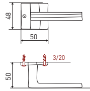
béquille sur rosace Rayure
