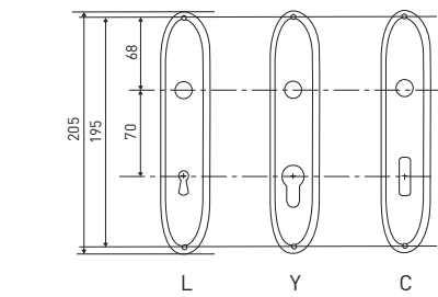
béquille sur plaque Acine
