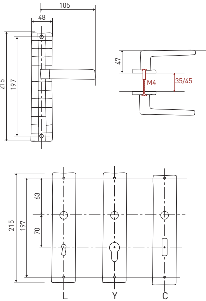
béquille sur plaque Caro
