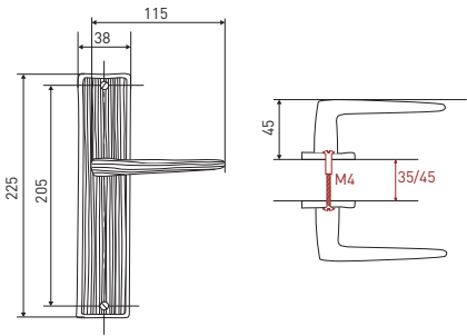
béquille sur plaque Écorce
