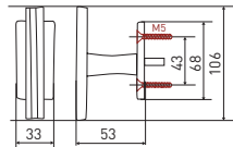
poignée de fenêtre Rayure
