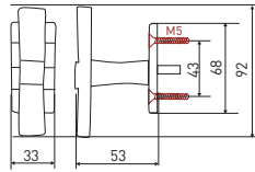
poignée de fenêtre Caro
