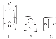
entrée de serrure Cubist
