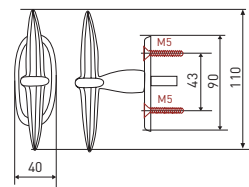
poignée de fenêtre Fuso
