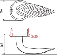
béquille sur rosace Acine
