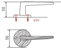
béquille sur rosace Écorce
