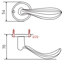
béquille sur rosace Plissé
