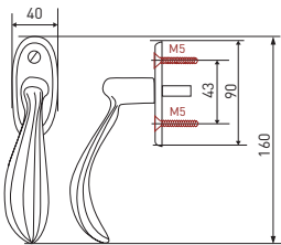
poignée de fenêtre Plissé
