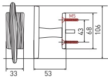
poignée de fenêtre Écorce
