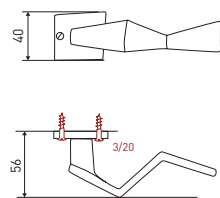
béquille sur rosace Cubist
