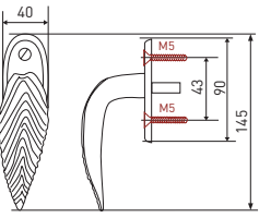
poignée de fenêtre Acine
